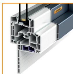
Sanierungs-Blendrahmen
