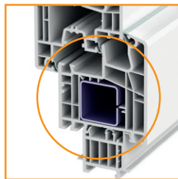
ERGOLINE-S mit Stahl im Blendrahmen
