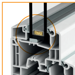
Glasabstandhalter
